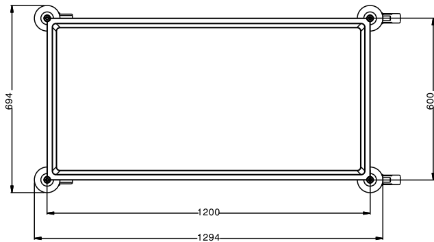
Boven aanzicht
